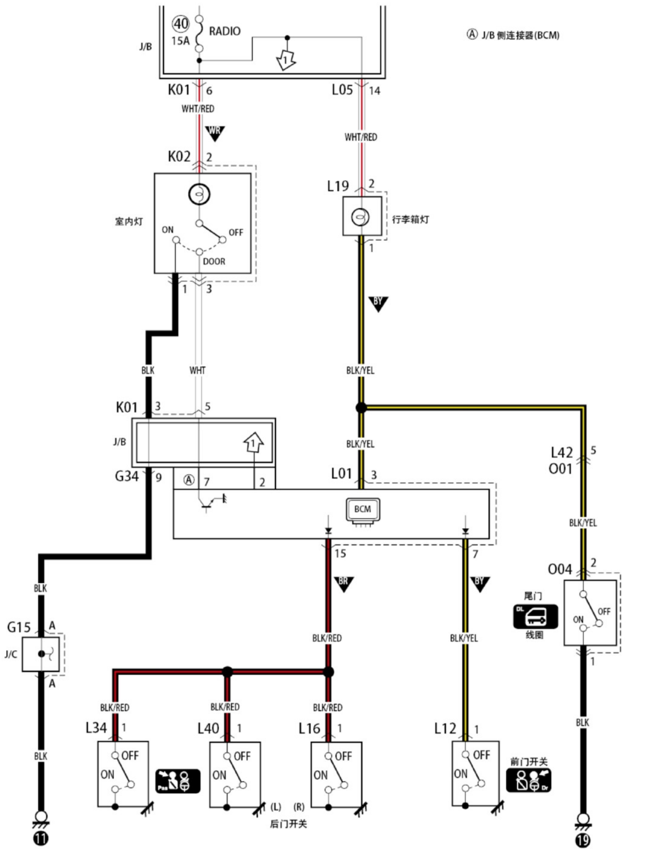
D-5内部照明系统线路图
