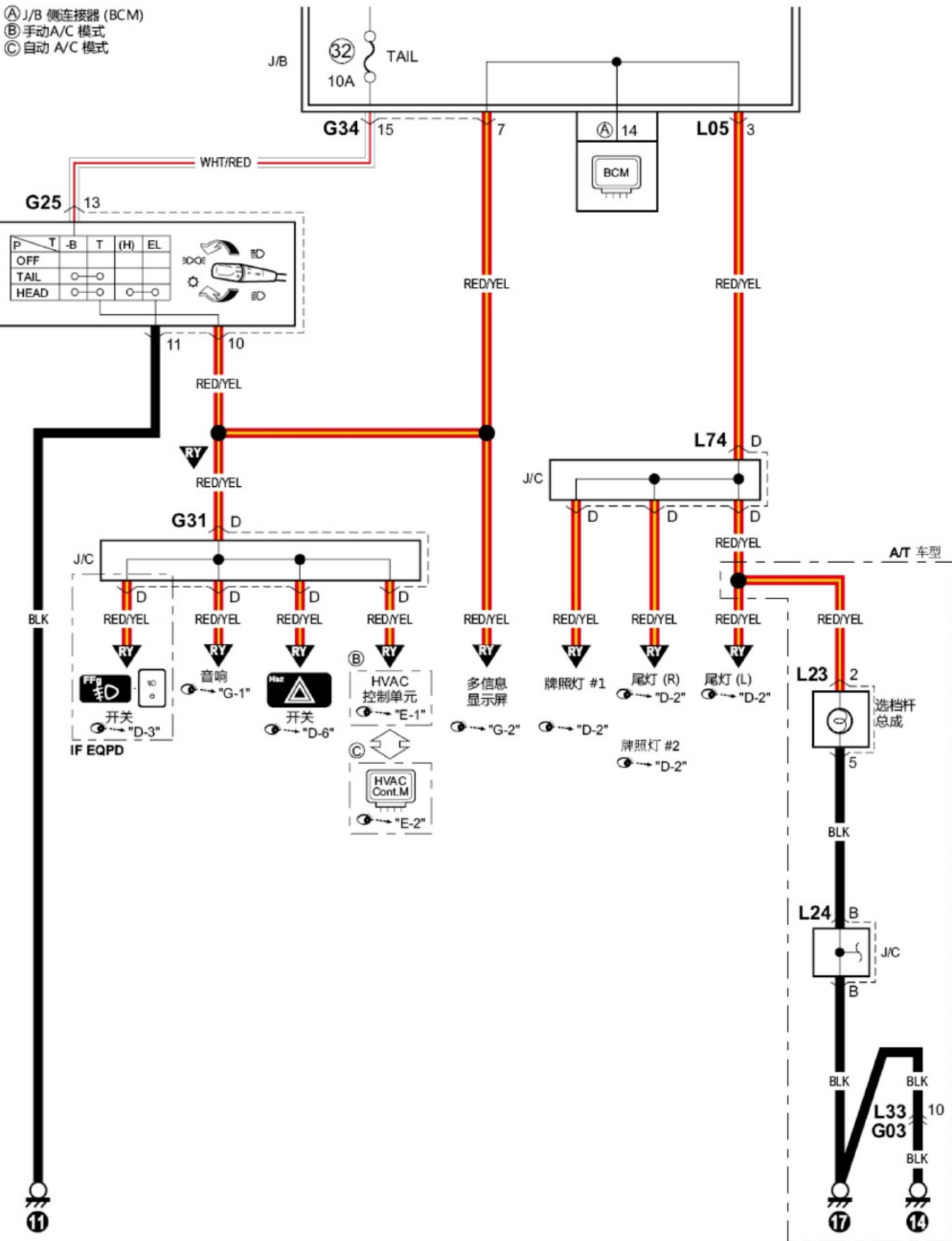
D-4照明灯系统线路图
